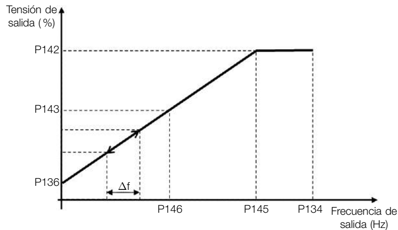
Figura 8.17: Compensación de deslizamiento en un punto de operación de la curva V/f
