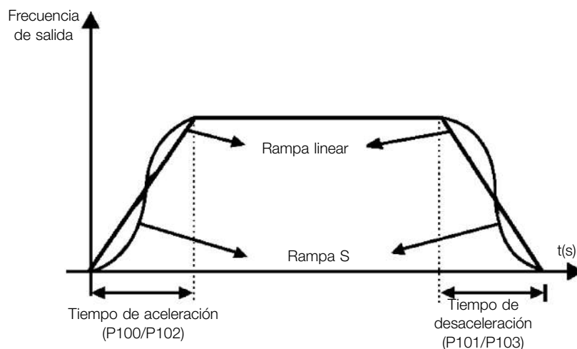
Figura 8.1: Rampa S o rampa linear
