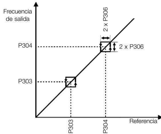
Figura 8.10: Actuación de la frecuencia evitada
